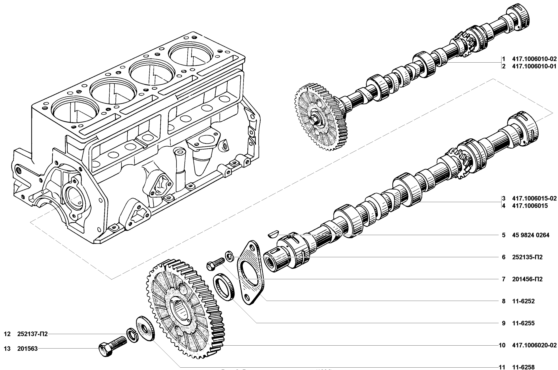
Рис. 8. Вал распределительный (1006) Fig. 8. Camshaft (1006)
